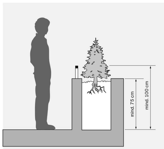
Abbildung 7 Geländer - Pflanzentrog
