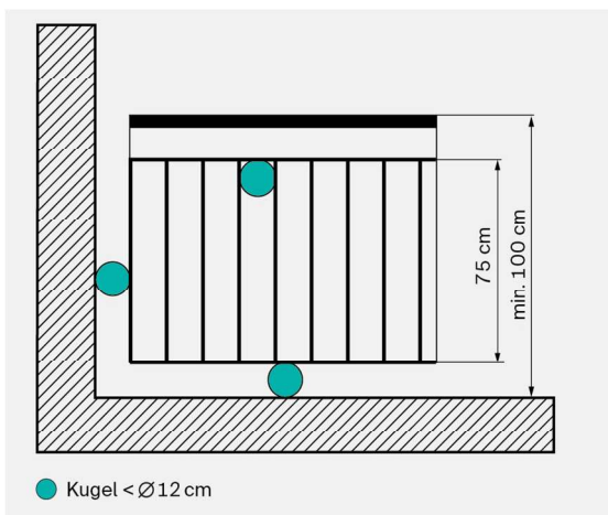
Abbildung 9 Geländer - Staketten
