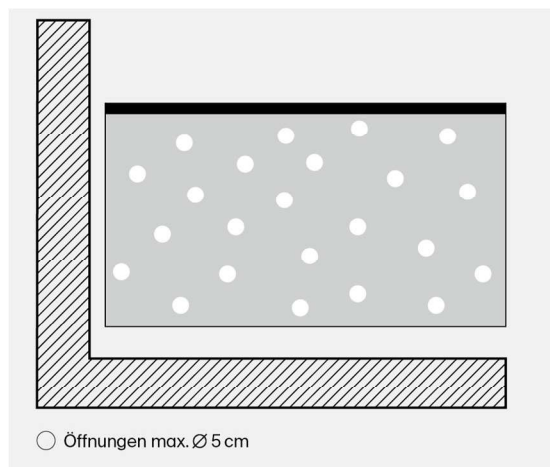
Abbildung 11 Geländer - Füllungen
