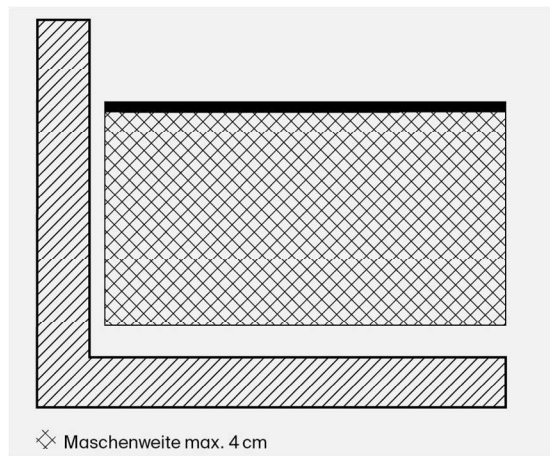
Abbildung 10 Geländer - Füllungen
